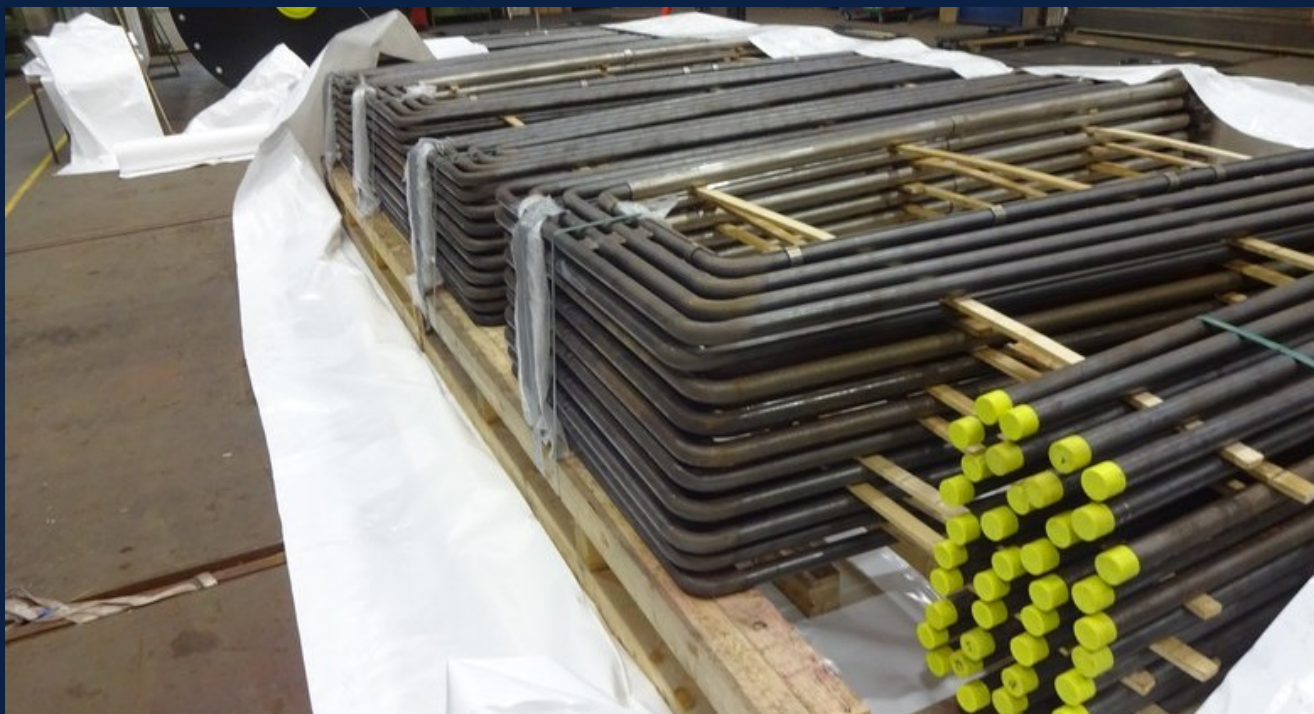
Serpentins de surchauffeur · ROHRLINE
